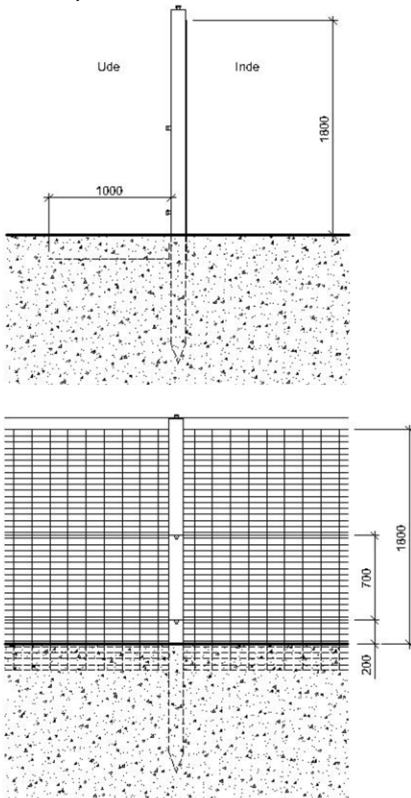
Figur 2. Forslag til opbygning af rovdyrhegn
